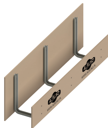
ALRUNO SZALUNEK TRĄCONY DO STROPU Z USKOKIEM D201
