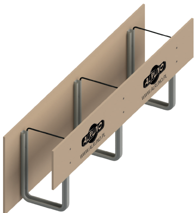
ALRUNO SZALUNEK TRĄCONY DO STROPU Z USKOKIEM D200
