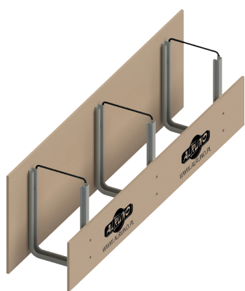
ALRUNO SZALUNEK TRĄCONY DO STROPU Z USKOKIEM D202
